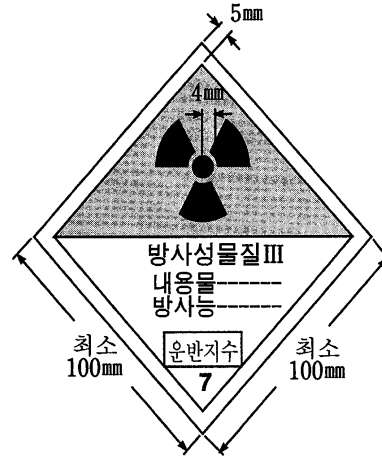
[부표 4] 제3종 황색운반표지
