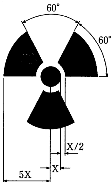
[부표 1] 방사능표지의 규격
