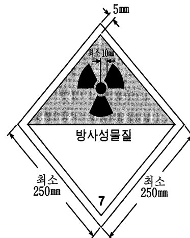
[부표 4] 제3종 황색운반표지
